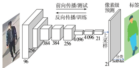
图 8 语义分割模型 FCN
